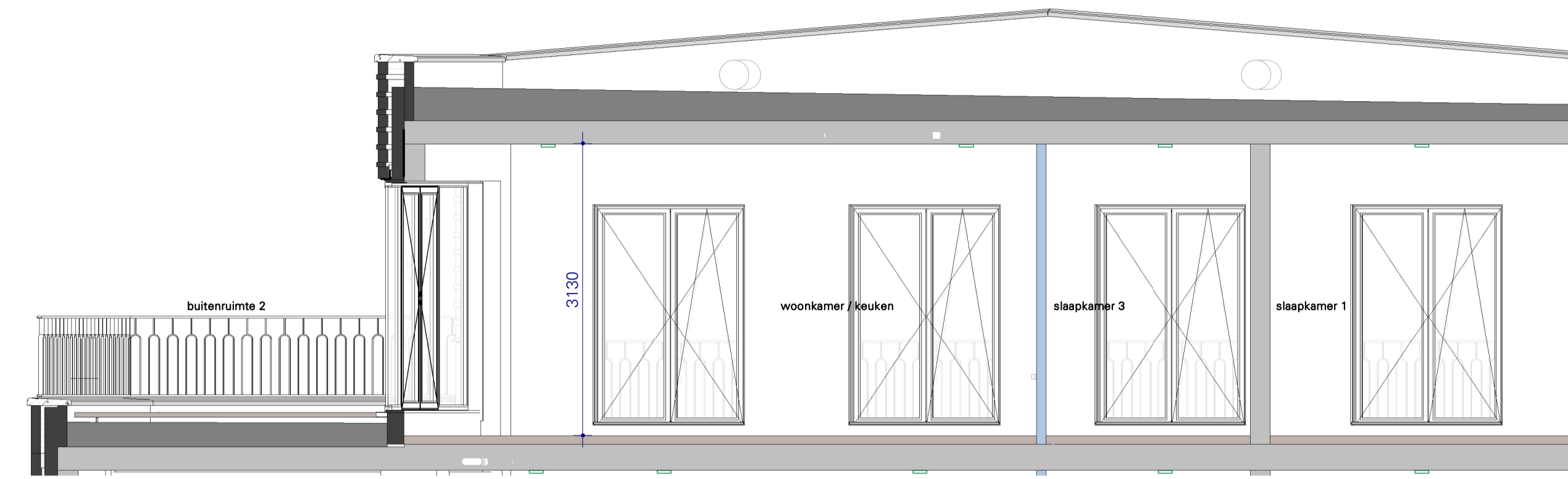
VK Doorsnede B - Blok E -bnr076
