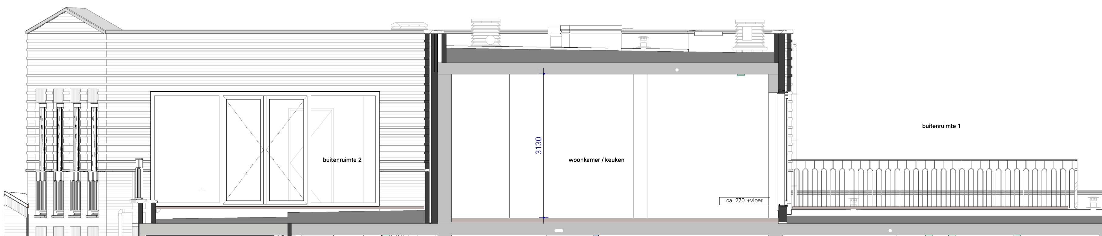
VK Doorsnede A - Blok E -bnr076
